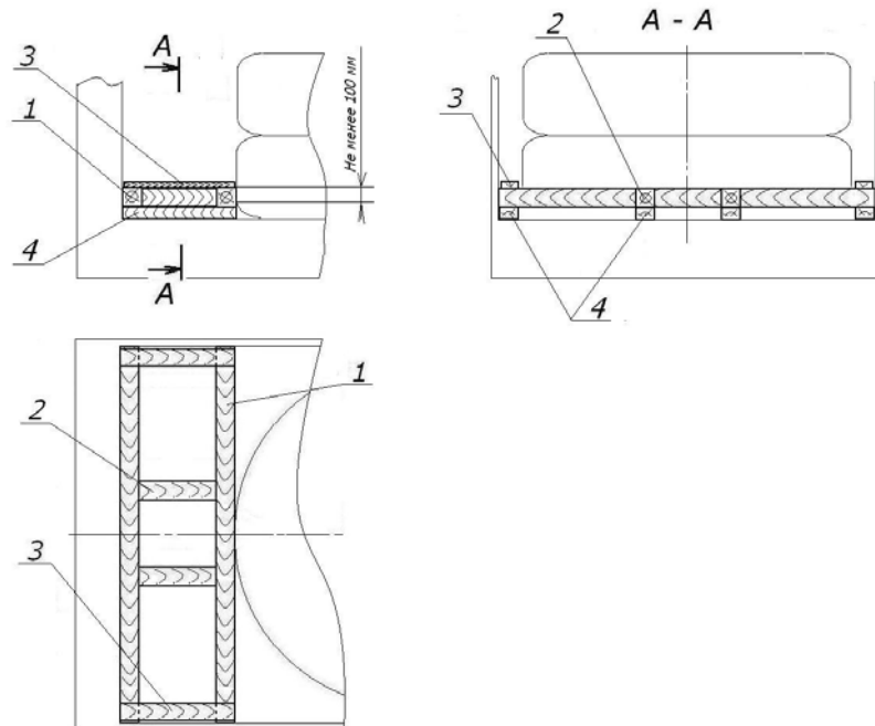
Рисунок 17 – Распорная рама
