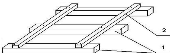
Рисунок 52 1 – распорный брусок; 2 – соединительная планка
