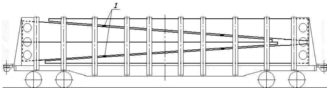
Рисунок 92 1 – прокладка
