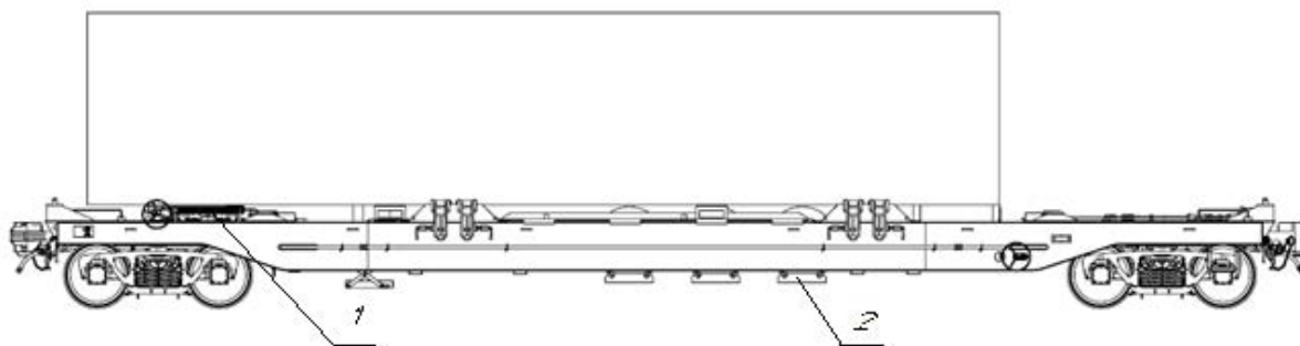
Рисунок 22 – Размещение и крепление полуприцепа 1 – седельное устройство; 2 – съемное многооборотное средство крепления
