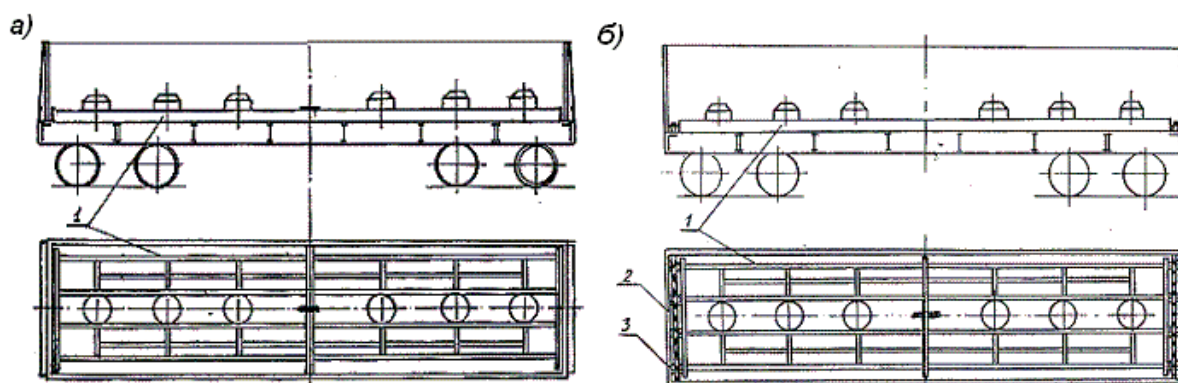
Рисунок 257 – Размещение комплекта поддонов в полувагоне: а – длиной кузова до 12228 мм включительно; б – длиной кузова свыше 12228 мм 1 – поддон; 2 – скрепляющая доска; 3 – распорный брусок
