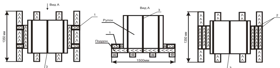
Рисунок 323 1 – продольный брусок; 2 – набор поперечных брусков; 3 – металлическая лента Рулоны в полувагоне размещают:
