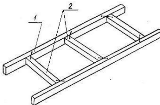
Рисунок 51 1 – упорный брусок; 2 – распорный брусок
