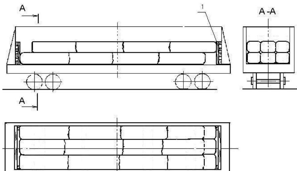
Рисунок 17 1 – торцевой щит
