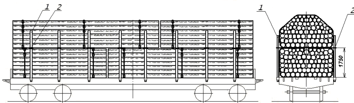
Рисунок 24 1 – стойка; 2 – стяжка
